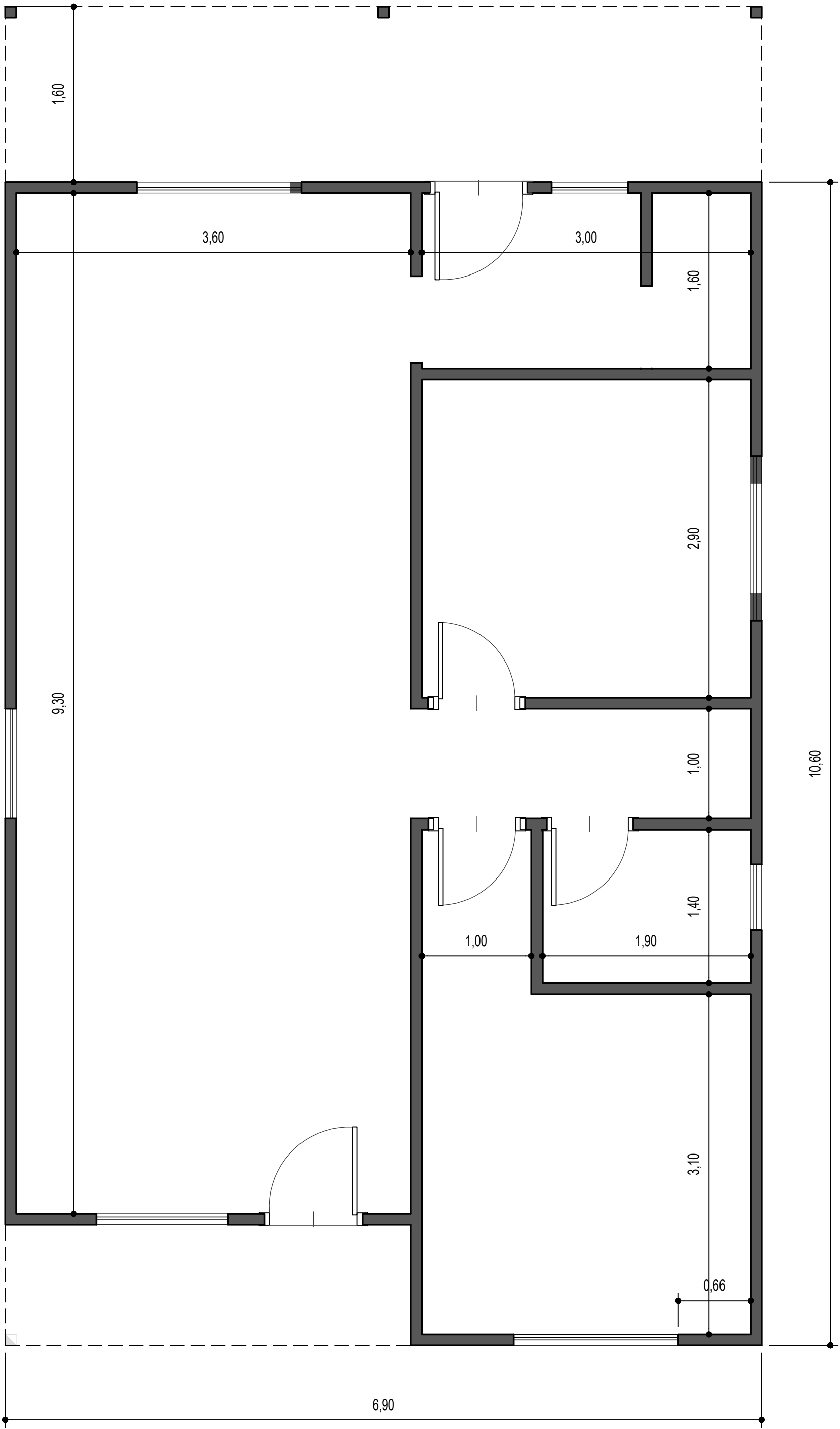
PLANTA ACOTADA
